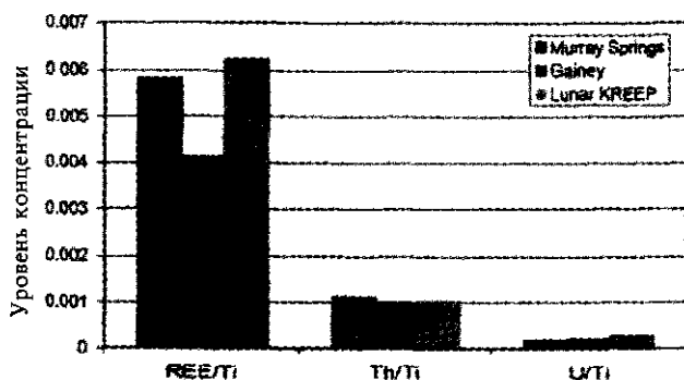
KREEP магнитных частиц эпохи кловис в сравнении с KREEP лунных образцов
