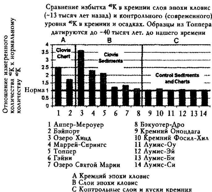
Илл. 25.7. Сравнение избытка ^{40}\text{K} в кремнии слоя эпохи кловис и осадках и современного уровня в кремнии и осадках. Все образцы датируются временем ~13 тысяч лет назад, кроме образца из Топпера, который относится, похоже, ко времени ударной волны 32 тысяч лет назад. Все образцы эпохи кловис показывают повышенное количество ^{40}\text{K} .
