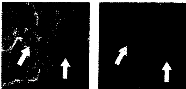
Илл. 4.9. Фотография и соответствующий ей снимок в рентгеновских лучах двух частиц. Одна частица видна, другая не видна, но от нее есть ямка. Это предполагает, что оба пятна появились одним и тем же образом
