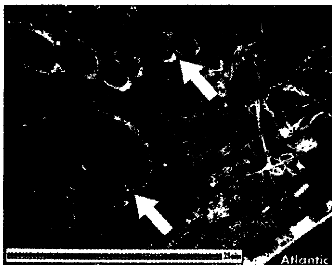
Илл. 10.2. Это фото с воздуха Миртл-Бич, Южная Каролина, показывает кластеры пересекающихся «заливов» (показаны стрелками), которые обычно выглядят на земле как болота с невысокими краями. Источник: Американская геодезическая служба
