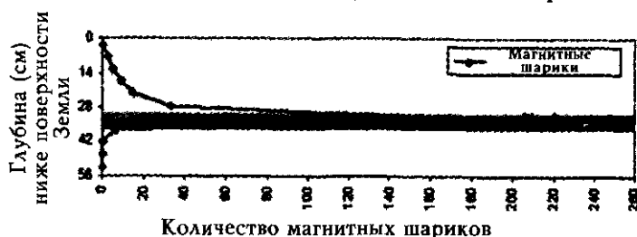
Илл. 2.9. Магнитные сферы из Гэйни. Большинство слоев почти не содержат магнитных сфер. Большая часть сфер находится в слое эпохи кловис
