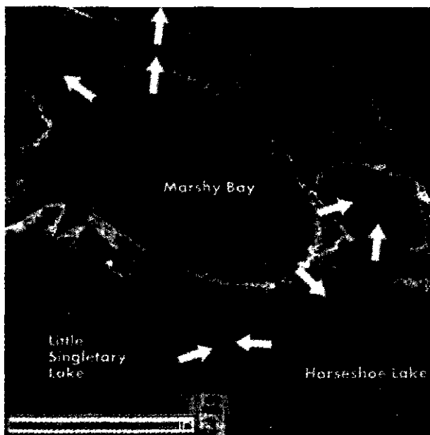
Илл. 17.1. «Залив» Марши и кластер «заливов» в Северной Каролине с перекрывающимися приподнятыми краями. Стрелки показывают места, где более поздний «залив» перекрывает более ранний. Из одиннадцати «заливов» десять перекрывают другие или сами являются перекрытыми. Ветер и вода не могут создать такой эффект, в то время как при столкновении с космическим телом это возможно. Получено из Геодетической службы США
