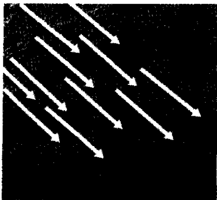
Илл. 19.1. Вдоль границы Северной и Южной Каролины Дуг Джонсон измерил направление по компасу в одиннадцати округах. Все оси оказались параллельными и шли с северо-запада. По Д.В. Джонсону (1942)
