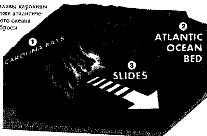
Илл. 33.2. Восточный берег, показывающий размещение самых больших подводных сбросов непосредственно у берегов «заливов Каролины».
