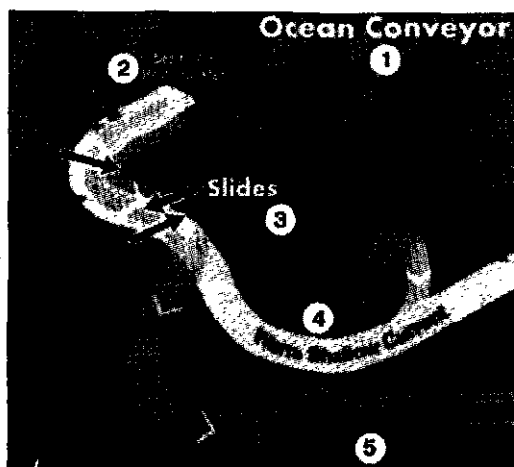
Илл. 33.7. Петлеобразные полосы «океанского конвейера» проходят прямо через главные места сбросов, указанных стрелками. Источник: Эн-Оу-Эй-Эй
