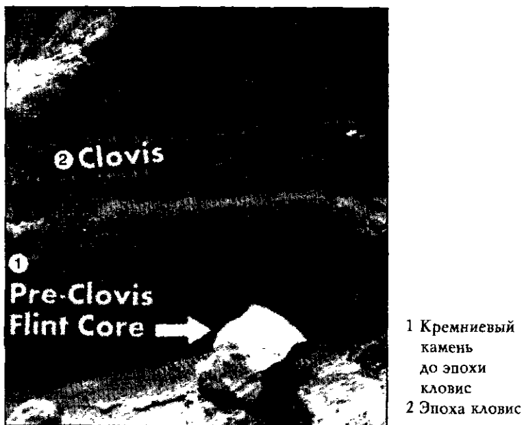
Илл. 9.3. «Нижнее место раскопок». Точки показывают уровень эпохи кловис, а стрелка указывает на большой кремниевый камень до эпохи кловис. Обработчик камня сидел здесь, отрубая кремниевые сколы, которые он использовал для изготовления других орудий труда
