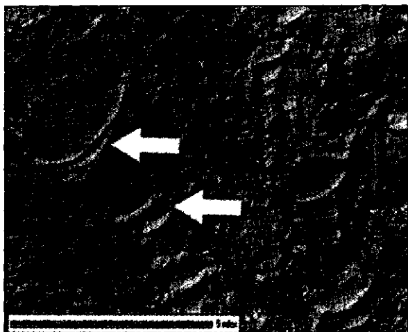
Илл. 20.1. Обработанное на компьютере изображение «дождевого бассейна» в округе Гранд, Небраска, показывающее многочисленные перекрывающиеся участки, которые выглядят точно так же, как «заливы Каролины».
