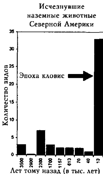
Илл. 1.2. Число исчезнувших в эпоху кловис видов сравнимо с числом исчезнувших видов за предыдущие 3,5 миллиона лет. Данные из Martin (1984)
