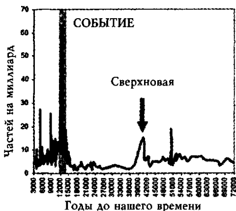
Илл. 30.3. Произошло внезапное резкое увеличение количества аммиака во время столкновения. Данные по Легранду и Де Ангелису (1995)
