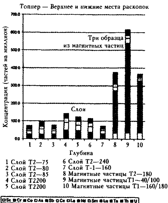
Илл. 25.4. Сравнение КРЕЕР в магнитных частицах с КРЕЕР в разных слоях на месте раскопок эпохи кловис в Южной Каролине. КРЕЕР существенно выше в магнитных частицах.
