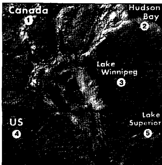
Илл.31.1. Это обработанное на компьютере изображение показывает западные равнины Канады и Соединенных Штатов. Заметьте, как движение ледника и талой воды прорезает отчетливо видимые желобки на земле, которые простираются через весь континент на протяжении нескольких тысяч миль.
