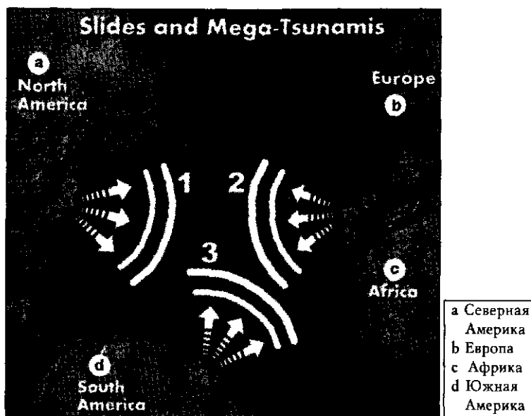
Илл. 33.5 Предполагаемая нами последовательность событий, связанных с цунами. Сначала произошли сбросы 1, вызвав цунами, которые привели к сбросам 2. Все это, возможно, случилось за двадцать четыре часа.
