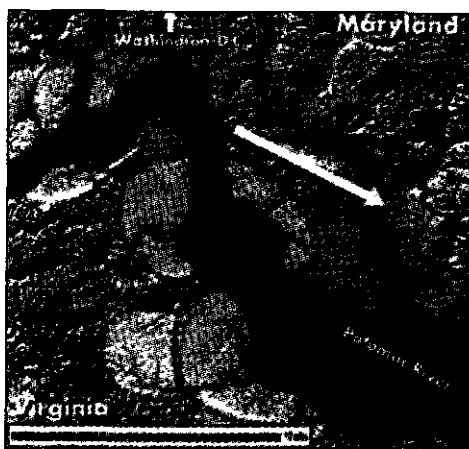
Илл. 19.5. Обработанная на компьютере фотография показывает почти точную ориентацию «восток-запад» некоторых предполагаемых «заливов» вдоль реки Потомак, в нескольких милях к востоку от Фредериксбурга и примерно в тридцати милях к югу от Вашингтона. Самый большой «залив» имеет примерно девять миль в длину, занимая всю ширину реки и врезаюсь в берега Виргинии и Мэриленда.
