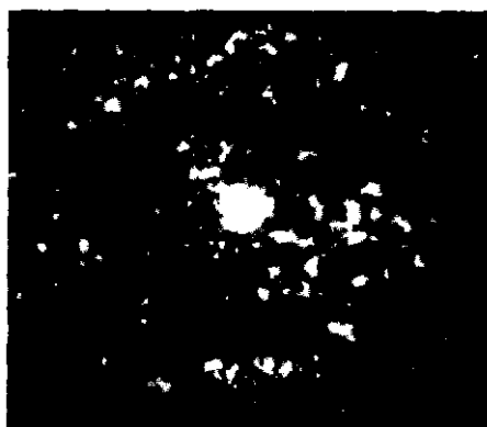
Илл. 14.2. Т Pyxidis, взорвавшийся «карлик», сформировавший тысячи огромных комков вещества, а не расширяющуюся гладкую оболочку ( bubblesite.org/newscenter/newsdesk/archive/releases/1997/29 ). Источники: Шара, Уильямс и Зарек (Научный институт космических телескопов); Джилмоззи (Европейская южная обсерватория); Пряльник (Университет Тель-Авива) и НАСА
