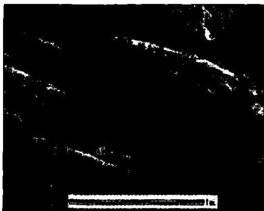
Илл. 8.2. Воздушное фото геологической съемки США. Поля друмлинов около Поуерса, Мичиган. Длинные веретенообразные фигуры типичны для этих земляных образований ледникового периода
