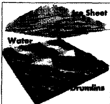
Илл. 8.3. Мы «наклонили» ледник, чтобы показать, как образуются друмлины. Ледниковая талая вода, проникая между ледником и землей, создает друмлины. По Шоу и Джилберту (1990)
