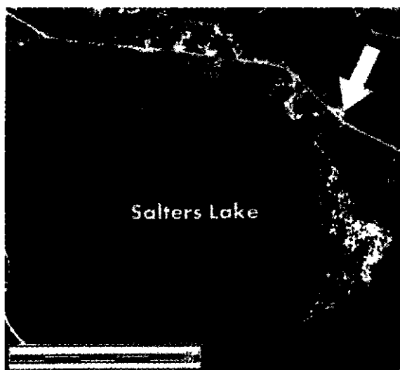
Илл. 10.5. Стрелка указывает на северо-восточный берег озера Солтерс, где я взял первые образцы. Заметьте яркий белый край из песка, который содержит столь мало питательных веществ, что на нем ничего не растет.
