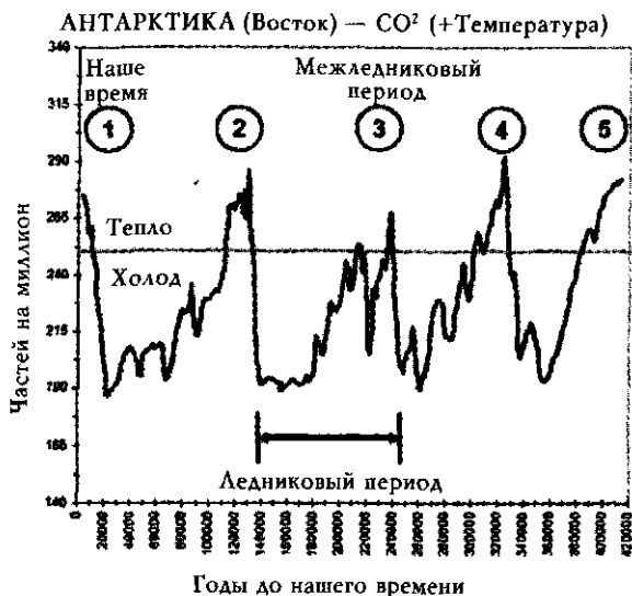
Илл. 2.3. Ледниковые периоды по содержанию CO 2 на станции Восток, Антарктика. Этот график «покрывает» последние 420 тысяч лет и показывает четыре последовательных ледниковых периода, каждый из которых продолжался 100 тысяч лет. В настоящее время Земля находится в коротком межледниковом периоде, как можно видеть по пяти резким пикам. После каждого пика холод возвращается. Данные из Петит, Эн-Си-Ди-Си
