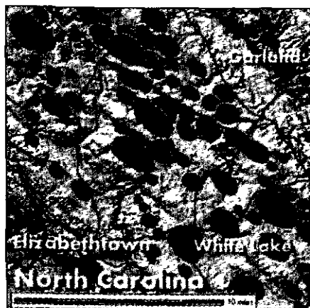
Илл. 10.4. «Трехмерная цифровая модель» показывает кластеры из сотен заливов Каролины в округе Блэден, Северная Каролина. Заметьте, что многие «заливы» пересекают границы соседних «заливов».
