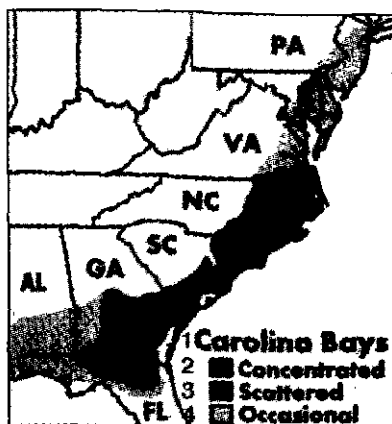
Илл. 10.3. «Заливы» протянулись от Алабамы до штата Нью-Йорк. Данные от Проути (1952)
