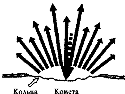
Илл. 27.5. Столкновение с легкой кометой направляет много энергии вверх в атмосферу и оказывает слабый эффект на материковую породу, образуя неглубокий кратер. По О'Кифу и Эхренсу (1982)
