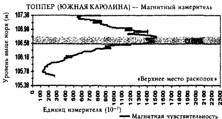
Илл. 9.2. Уровень намагниченности, как и число магнитных частиц, имеет максимальное значение в слое эпохи кловис
