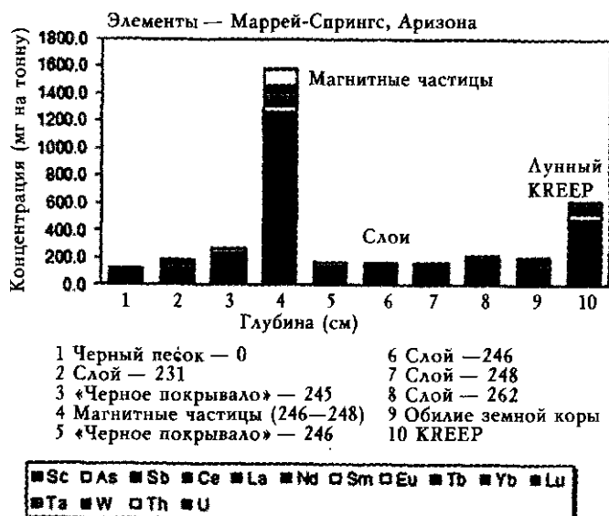
Илл. 25.3. Сравнение магнитных частиц в Маррей-Спрингс с данными по слоям на предмет содержания редких элементов
