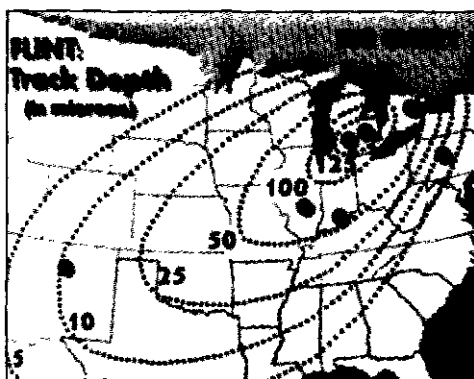
Илл. 1.5. Глубина выбоин в образцах кремния эпохи кловис. Глубина уменьшается по мере удаления от Великих озер, что заставляет предполагать, что именно этот район был местом «События»
