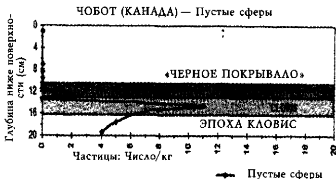
Илл. 6.3. Большой пик в количестве пустых частиц на уровне эпохи кловис
