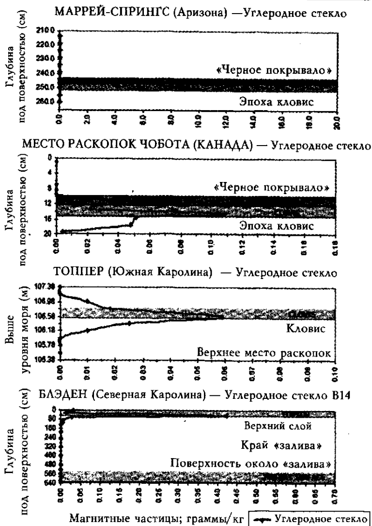
Илл. 34.5. Этот обобщенный график показывает, что пики в стеклообразном углероде почти идентичны на главных местах раскопок эпохи кловис в Маррей-Спрингс, Чоботе, Топпере и «заливе Каролины» в округе Блэден
