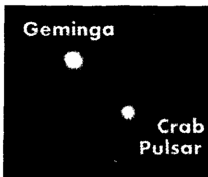
Илл. 15.2. Является ли это действительным изображением убийцы? На фотографии видны два остатка сверхновой — пульсары Краб (справа) и Геминга (слева). Геминга является нашим кандидатом на статус «автора» «События».
