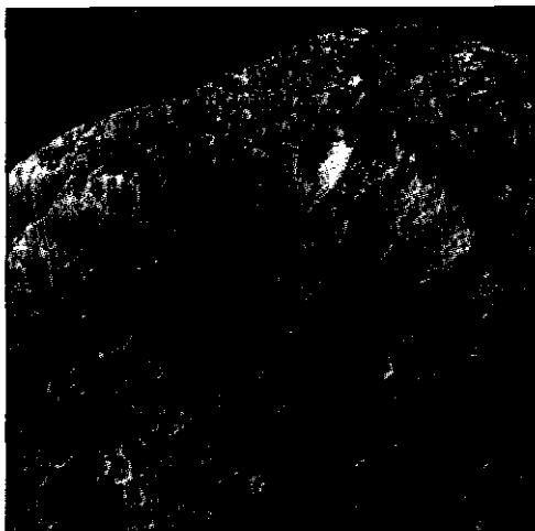
Илл. 27.3. Эта фотография показывает имеющий низкую плотность Гиперион, спутник Сатурна, составляющий 155 миль в длину. Необычный вид и быстрое вращение показывают, что это — похожий на губку объект из скальной породы. Источники: Кассини Имидж Тим, Институт космических наук, лаборатория реактивного движения, Европейское космическое агентство, НАСА
