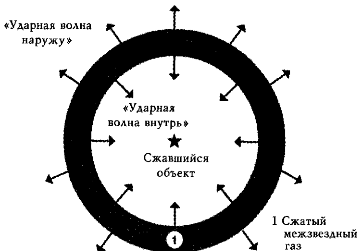
Илл. 14.1. «Ударные волны наружу» и «ударные волны внутрь» от сверхновой типа II создают нейтронную звезду или «черную дыру», в центре.
