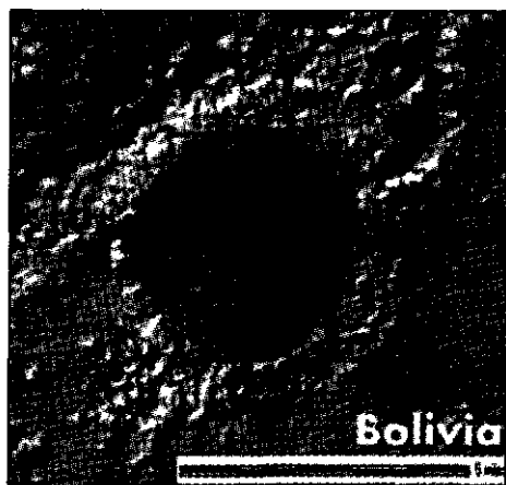
Илл. 29.1. Обработанное на компьютере изображение кратера в пять миль шириной. Источник: НАСА
