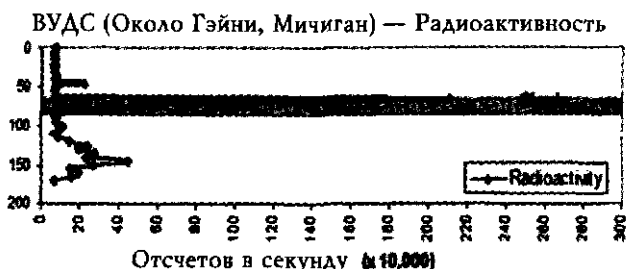
Илл. 2.1. Данные, взятые в Вудс-Сайт, показывают большой пик радиоактивности в слое эпохи кловис. Выше и ниже не видно почти ничего
