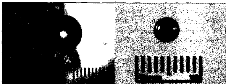
Илл. 2.8. Магнитная сфера из Гэйни. Другие частицы почти скрывают большую по размерам сферу (слева), которая имеет размеры почти в три раза большие, чем обычные частицы (справа). На фотографиях представлены сферы самых больших и самых малых размеров
