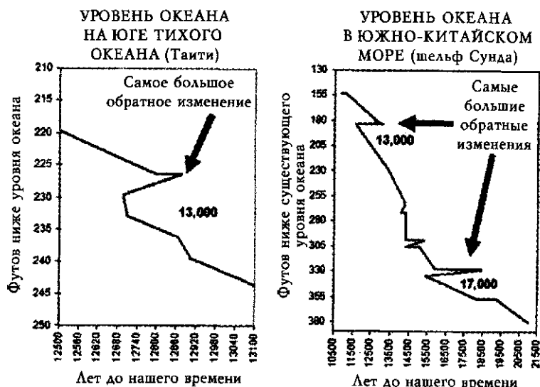
Илл. 32.4. Слева образцы с Таити показывают обратное изменение 13 тысяч лет назад: образцы из шахты могли бы показать обратное изменение 16 тысяч лет назад, но образцов столь давнего времени нет. Данные из: Бэрд и др. (1996). Справа образец с шельфа Сунда показывает два больших обратных изменения 13 и 17 тысяч лет назад. Данные по Хэнебуту и др. (2000)
