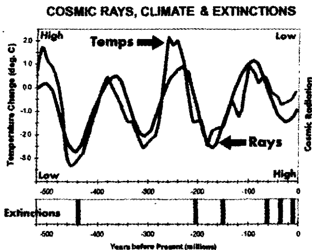
Илл. 16.2. Черная температурная линия, подсчитанная из космических потоков лучей, точно прослеживает существующий климат в течение последних 500 млн лет. Шесть из девяти последних затуханий также соединяются с увеличивающейся радиацией
