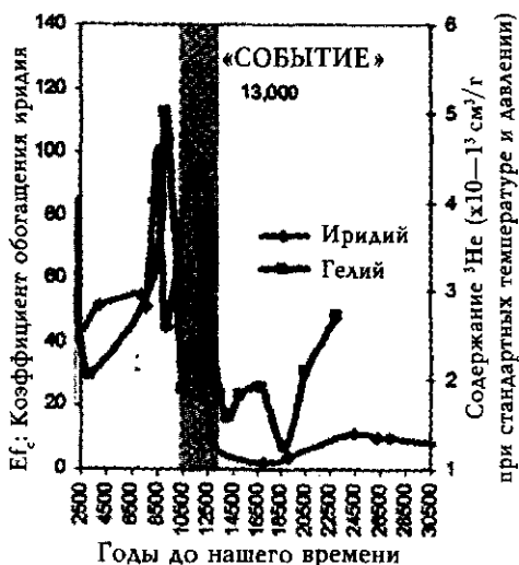
Илл.34.1. Примерно 13 тысяч лет назад гелий-3 и иридий имели большие пики концентрации — самые большие за 23 тысячи лет. Данные: по иридию из Габриелли, 2004; по гелию из Маркантонио, 2001
