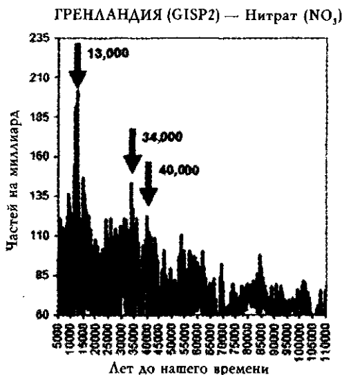
Илл. 16.3. Уровень нитрата из образца GISP2 из ледника в Гренландии. Заметьте, что во время «События» количество нитратов почти удвоилось и достигло максимума за последние 110 тысяч лет. Данные из: Маевский и др. (1997)
