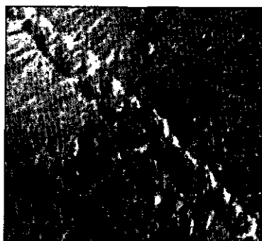
Илл. 18.2. Ганимед. Здесь показана почти идентичная картина на Ганимеде, одном из спутников Юпитера. Длинная цепь состоит из тринадцати отдельных перекрывающихся кратеров, которые НАСА считает образовавшимися от почти мгновенного столкновения в серии осколков комет. Источники: Проект Галилео, Университет Брауна, Лаборатория реактивных двигателей, НАСА
