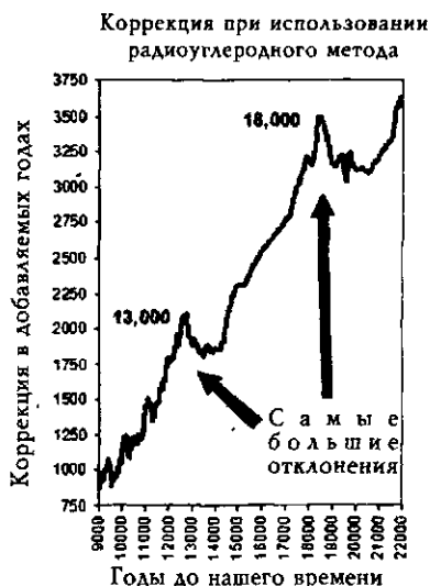
Илл. 1.4. Проблемы: непостоянное содержание ^{14}\text{C} и неверное отражение дат. Острые пики в 13 тысяч и 18 тысяч лет назад показывают, что какая-то причина увеличила содержание ^{14}\text{C} в окружающей среде. Данные из Reamer et al. (2004)
