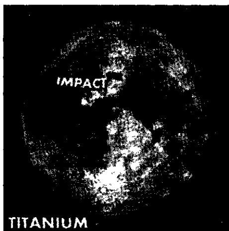
Илл. 25.1 Распределение титана на поверхности Луны. Это примерно те же районы, где есть железо, торий и калий, причем этих элементов почти нет на обратной стороне Луны. Получено от НАСА
