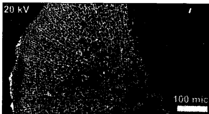
Илл. 34.3. Изображение, полученное в сканирующем электронном микроскопе, показывает подобную пыли структуру этой расколотой сферы. Вся сфера имеет примерно ту же ширину, что и человеческий волос
