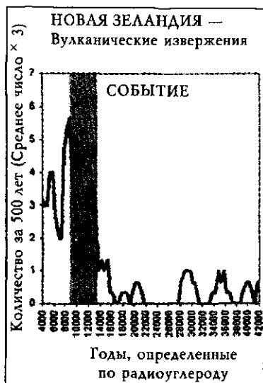
Илл. 30.2. Частота извержений внезапно увеличивается примерно 13—16 тысяч лет назад в Новой Зеландии, которая находится очень далеко от ближайшего ледника. Данные по Брисону (1988)
