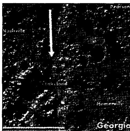
Илл. 19.4. Это созданное на компьютере изображение Геодезической службы США показывает место около Лэйкланда, Джорджия. «Заливы» в этом районе ориентированы почти точно на север, то есть в большей степени, чем было установлено Джонсоном раньше. Источник: Геодезическая служба США
