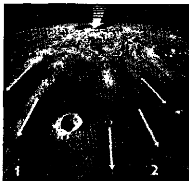
Илл. 18.3. Как формируются цепи. Когда астероид ударился о лунную поверхность много лет тому назад, это привело к образованию огромного кратера (в месте, показанном стрелкой вверху) и выброси-
