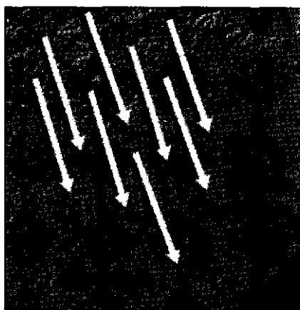
Илл. 19.3. Вдоль границы Джорджия — Южная Каролина Джонсон измерял направление осей «заливов» по компасу в восьми округах. Оси оказались направленными на северо—северо-запад. По Д.В.Джонсону (1942)
