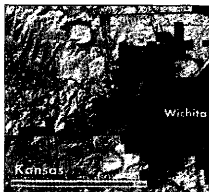
Илл. 20.2. Эта обработанная на компьютере фотография показывает кластер похожих на «заливы» «бассейнов» около Вичиты, некоторые находятся в пределах города.
