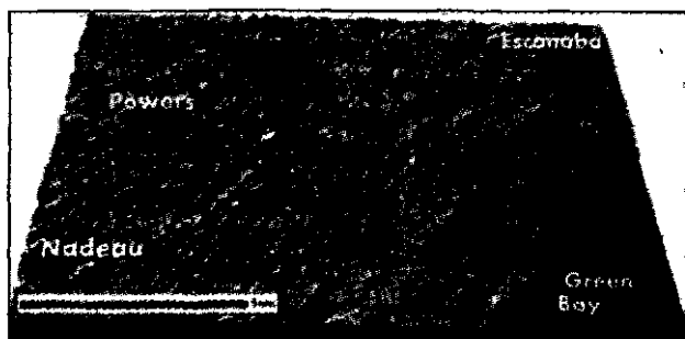
Илл. 8.4. На этом изображении — результат цифровой обработки фотографий геологической съемки США: видно поле с часто расположенными друмлинами в милю длиной, расположенное к западу от озера Мичиган около Эсканаба, Мичиган
