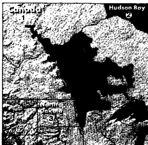
Илл. 31.3. Ледниковое озеро Агасси занимало большую часть Манитобы и часть Дакоты и Миннесоты. Оно было значительно больше, чем Верхнее озеро, видимое в нижнем правом углу.
