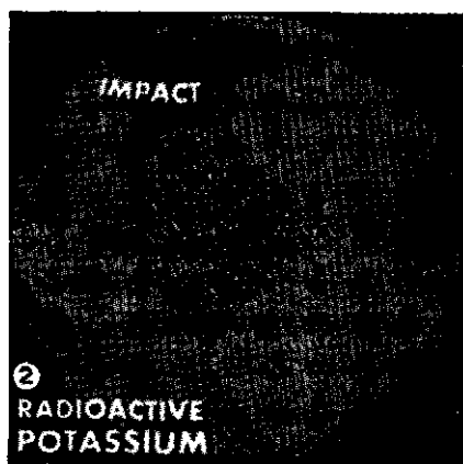
Илл. 24.5. Полученная со спутника «Одиссей» картинка радиоактивного калия в районах средних долгот Марса. Торий имеет тот же рисунок. Получено от НАСА/Джи-Пи-Эл/Университета Аризоны
