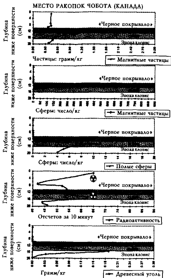
Илл. D.2. Основные маркирующие горизонты раскопок Чобот в Альберте. Стеклообразный углерод не показан, но он присутствовал в небольших количествах
