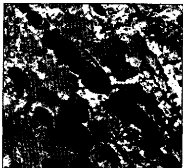
Илл. 18.1. Северная Каролина. Фото с воздуха «залива» Биш-Уайт и других «заливов» из длинной цепи тянущейся через округ Блэден. Эта цепь «заливов» имеет примерно двадцати пять миль в длину и более мили в ширину. Она, возможно, образовалась точно так же, как и цепи на Марсе и Луне, где их сформировали выбросы из основного кратера. Источник: Геодезическая служба США
