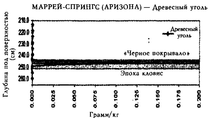
Илл. 3.7. Количество древесного угля максимально как раз в слое эпохи кловис, что заставляет думать, что в эту эпоху было много пожаров
