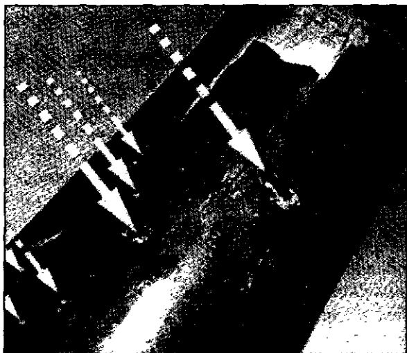
Илл. 4.7. Имеющий синий оттенок бивень из Сибири. Видны кратеры от семи магнитных частиц. Стрелки показывают направление движения. Самой длинной стрелой отмечен самый протяженный кратер, получившийся от наклонного удара. На других участках поверхности бивня кратеров нет
