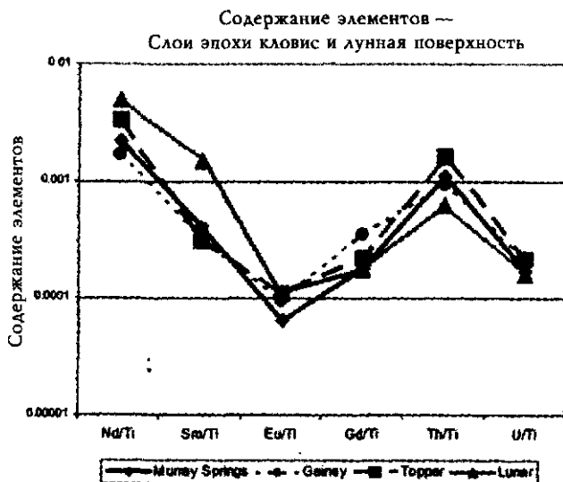
Илл. 25.2. Содержание различных редкоземельных элементов, а также тория и урана, с мест раскопок Топпер, Мэррей-Спрингс, Гэйни, а также с Луны, по сравнению с титаном
